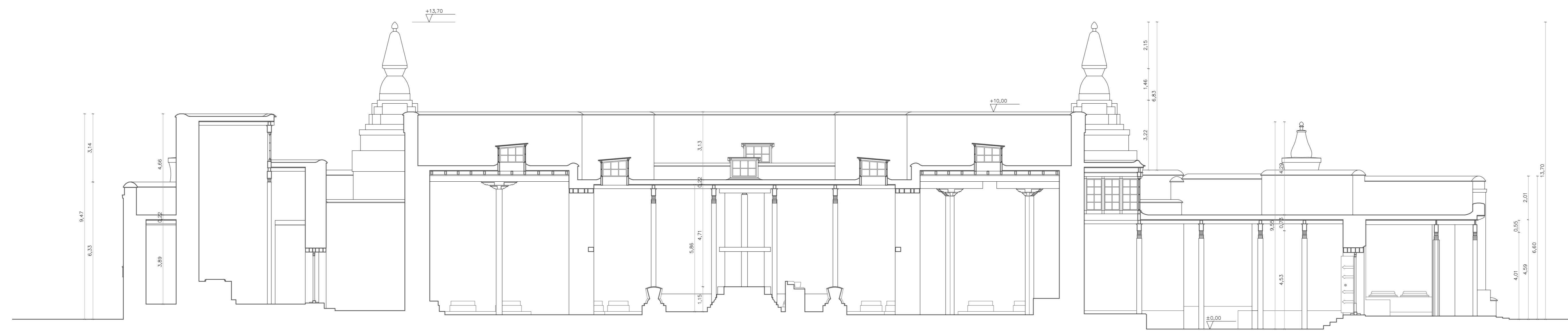
Longitudinal section A-A
