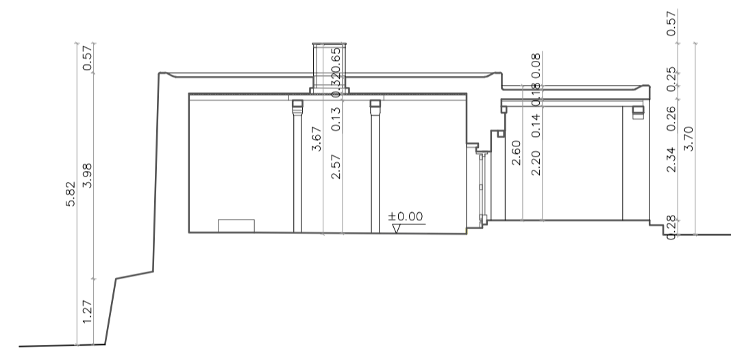
Longitudinal section A-A
